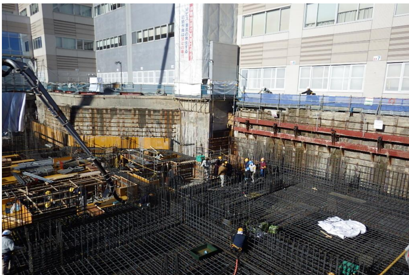
④ 耐圧盤2工区 マットスラブ下 コンクリート打設
